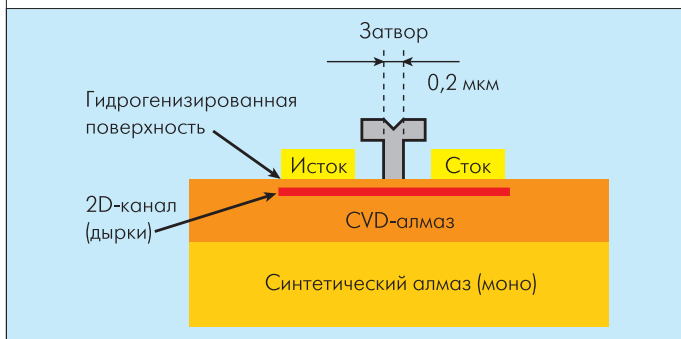
Рис. 11. Структура MESFET, выполненного на гидрогенизированной поверхности эпитаксиальной алмазной пленки
