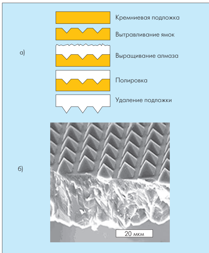
Рис.9. Принцип метода реплики (а) и массив алмазных пирамид (период 12 мкм), выращенных на анизотропно травленной кремниевой подложке (б)
