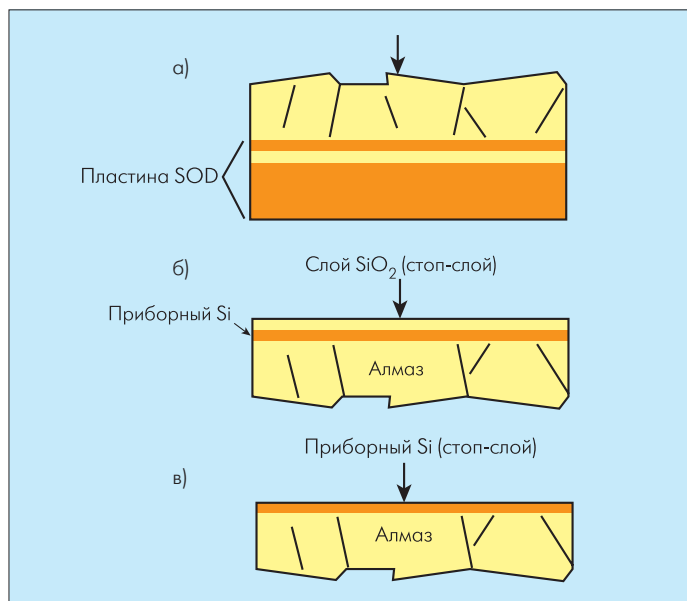
Рис. 10. Процесс изготовления SOD-пластины: а) осаждение пленки алмаза; б) травление Si в KOH; в) травление SiO 2 в HF [24]
