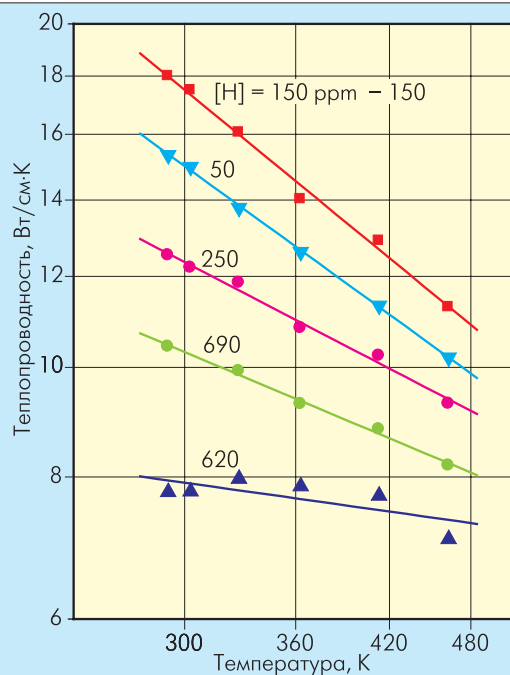
Рис.7. Температурные зависимости теплопроводности k_{||} в логарифмических координатах для алмазных пластин различного качества. Для каждого образца указана концентрация примесного водорода (ppm) [14]
